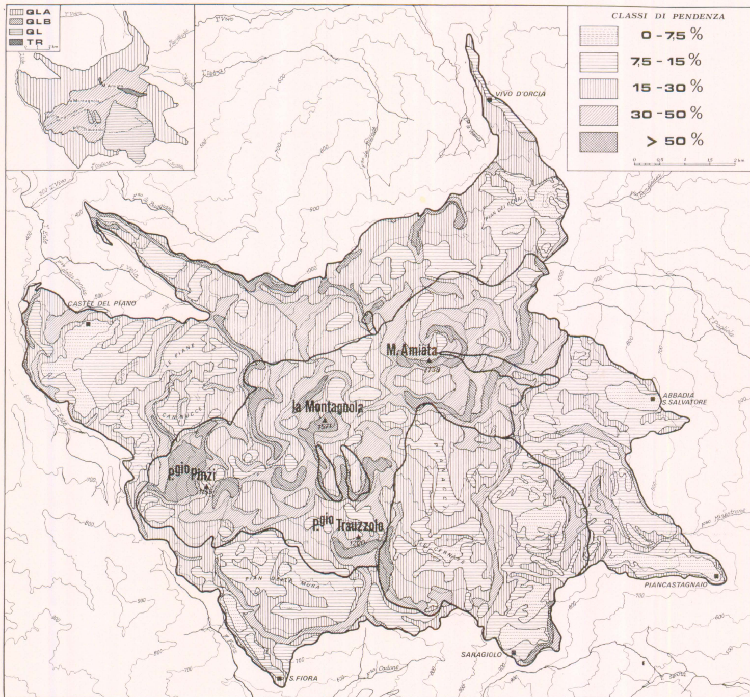
Fig. 2 - Carta delle acclività delle vulcaniti del Monte Amiata.
